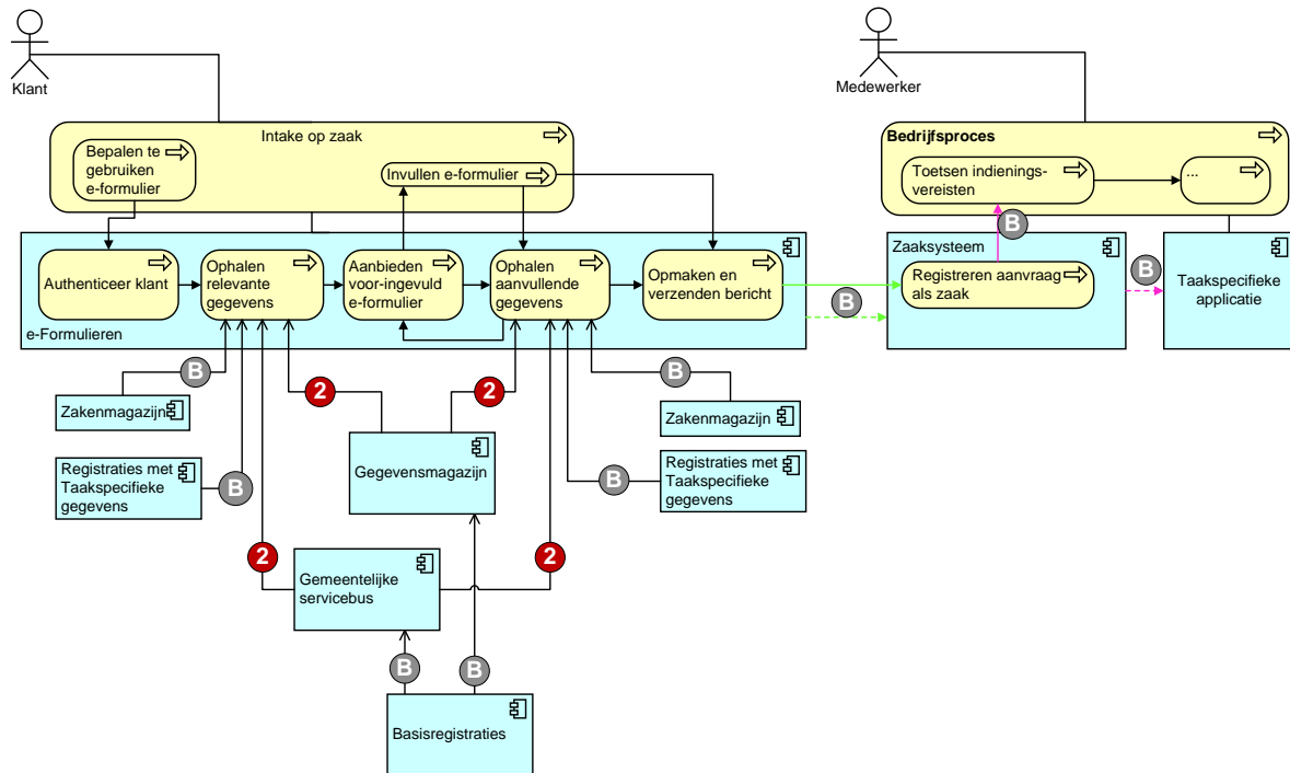
Figuur 5: Referentiearchitectuur
