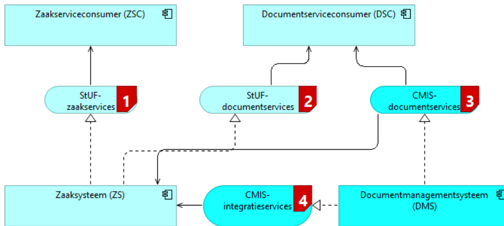
Figuur 5: Applicatiearchitectuur
